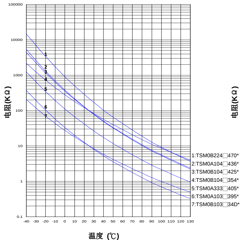
TSM0B103□34D* ~ TSM0B224□470*
