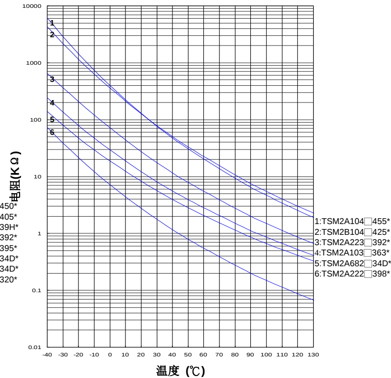
TSM2A222□398* ~ TSM2A104□455*
