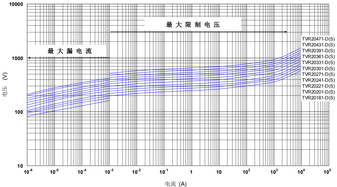
最大漏电流与最大限制电压曲线 (TVR20181-D(-S) to TVR20471-D(-S))
