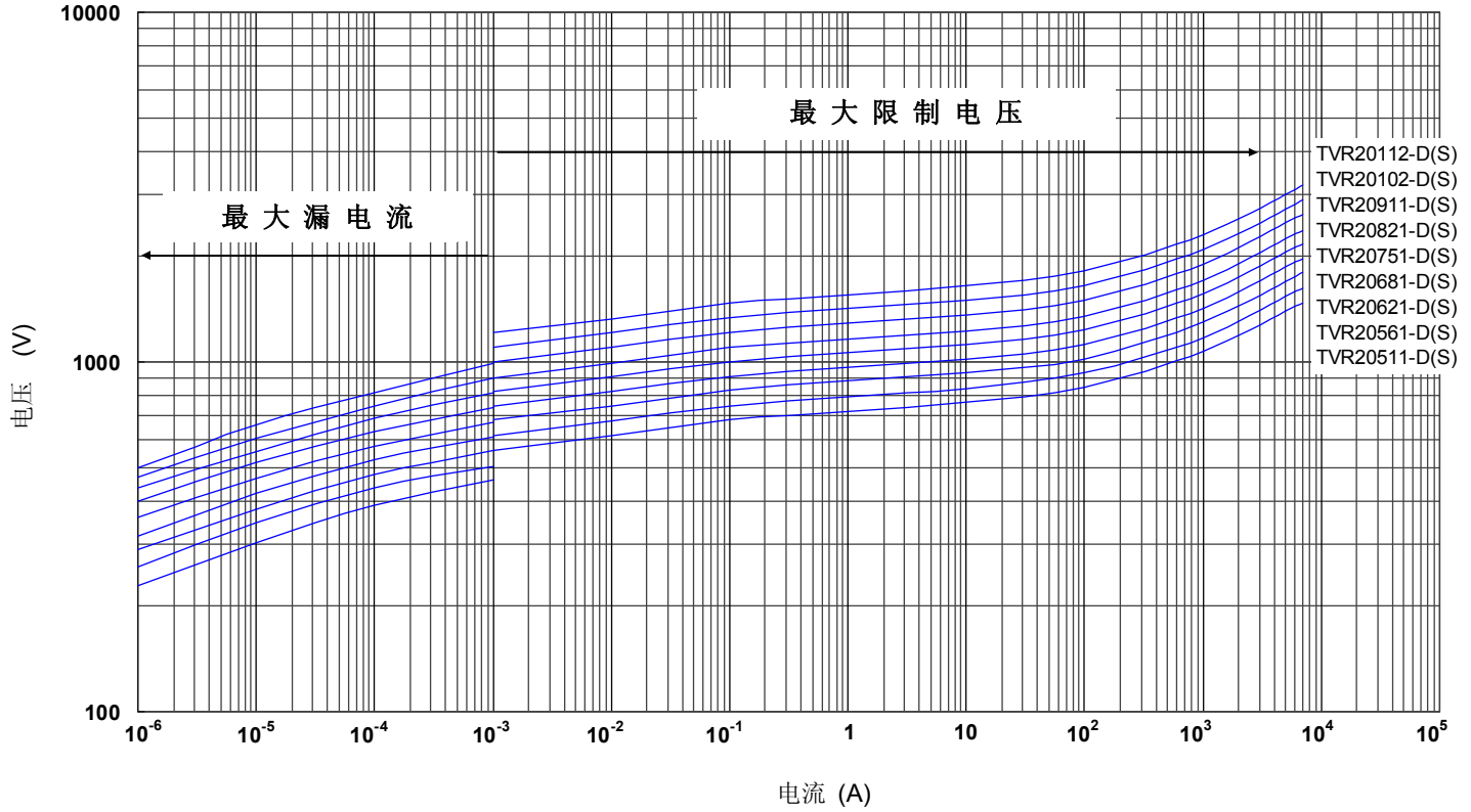
最大漏电流与最大限制电压曲线 (TVR20511-D(-S) to TVR20112-D(-S))
